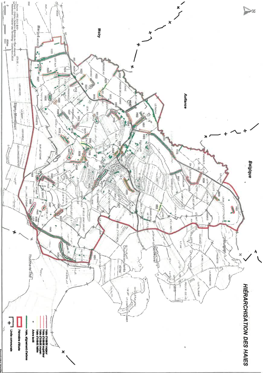
Carte n° 31 : Les haies
